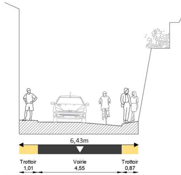
Coupe de l'existant sur la montée du Chemin Neuf
