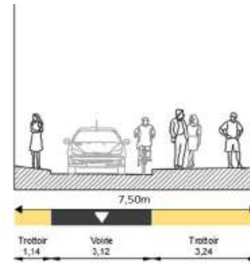
Coupe de l'existant sur la rue de Tramassac
