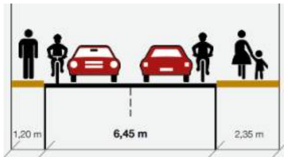
Profil existant rue de l'Antiquaille
